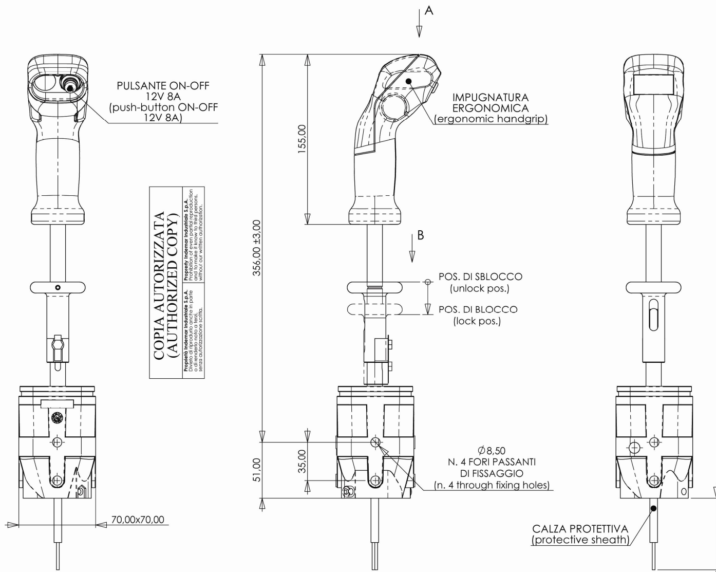
VISTA PARZIALE (partial view)
