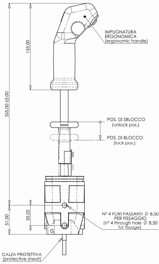
VISTA PARZIALE (partial view)
